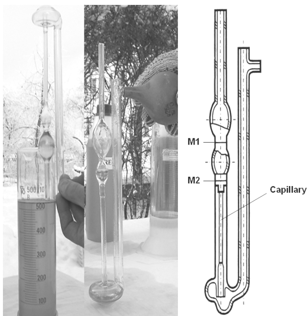
Fig. 1. Viscometer BИЖ-2 1 pav. Viskoizmetras BИЖ-2
